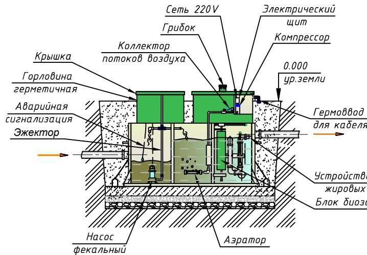
Разрез Б-Б
