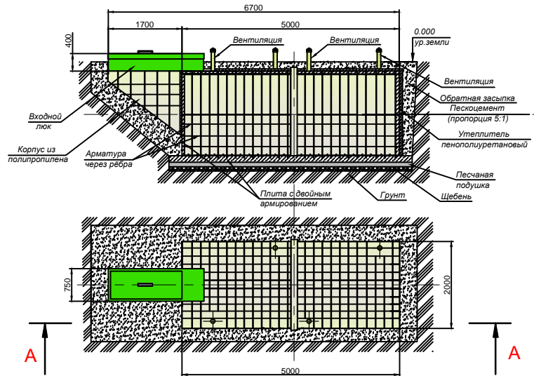
Разрез А-А
