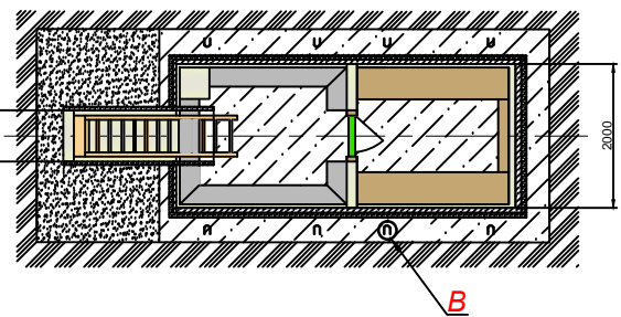
Разрез Б-Б
