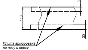
Г(1:5)
