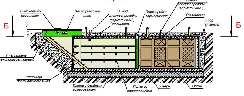
Разрез Б-Б
