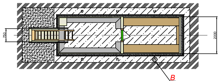
Разрез Б-Б
